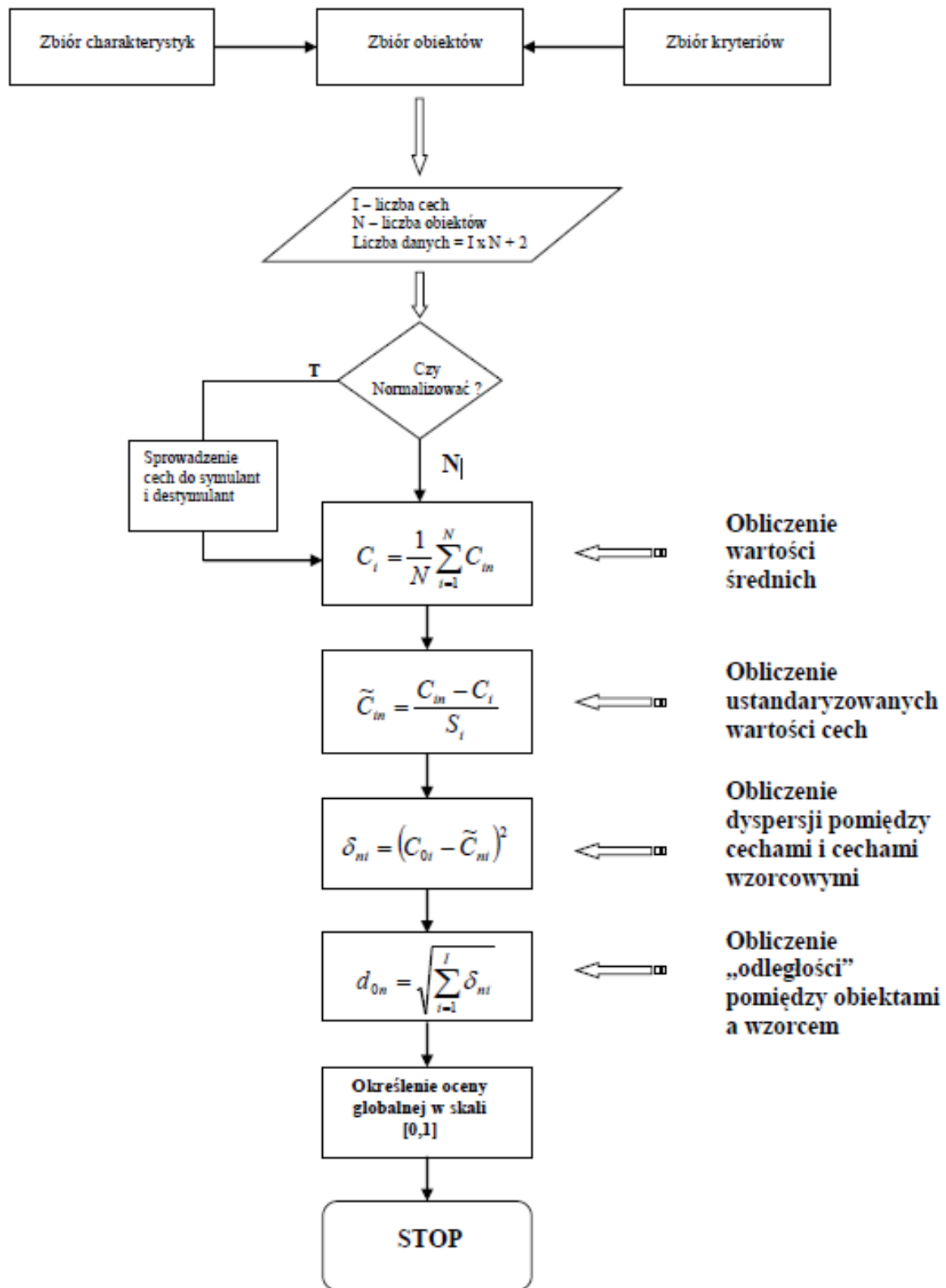
Rysunek 1. Algorytm metody taksonomii numerycznej
